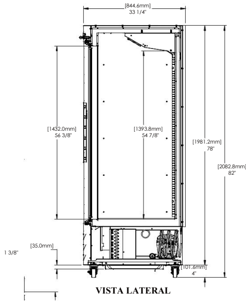
ELEVACIÓN
